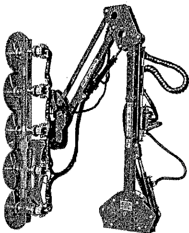
PJ 5 tárcsás síkfal metsző berendezés cikkszám: 15662110
