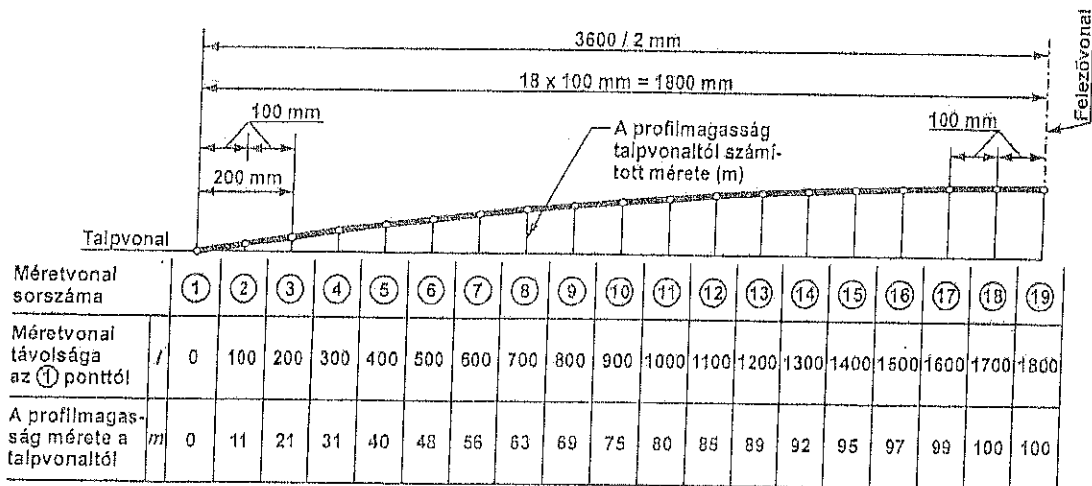
3. ábra – Íves keresztmetszetű menetdinamikai küszöb mintaszelvénye (arányrajz) és ellenőrző sablonjának méretei. (A méretek R=16 m sugarú küszöbök kitűzési adatai)
