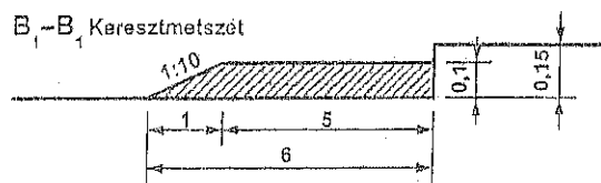
2. ábra – Pályaszintemelések geometriai kialakítása (ajánlott példák)
