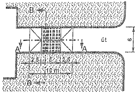
(B) Kiemelt szegélyek között, azokon túlnyúló lejtővel
