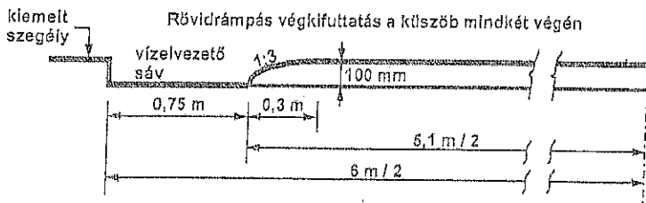
B-B Hosszmetszet
