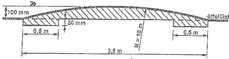
A-A Keresztmetszet
