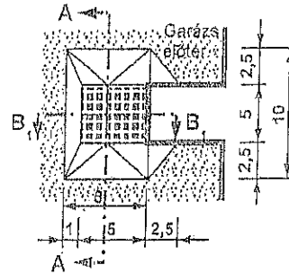
(C) Kiemelt és süllyesztett szegély között túlnyúló lejtővel és egyoldali hosszúrampás végkifuttatással.
