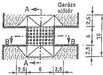
(B) Kiemelt szegélyek között, azokon túlnyúló lejtővel
