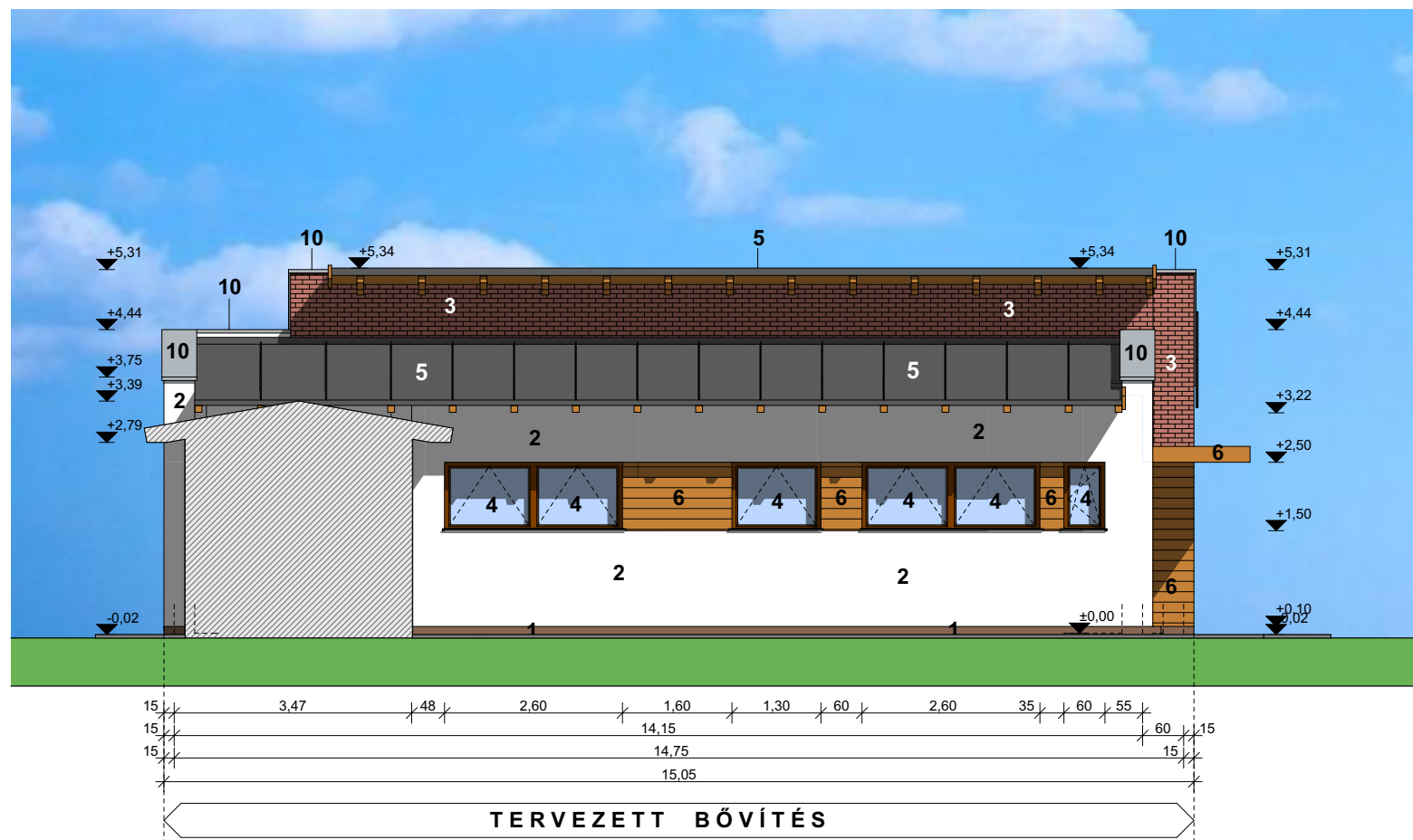
Tervezett BELSŐ UDVARI homlokzat
